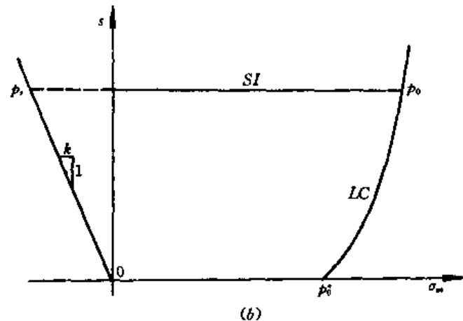
图 6-5 空间屈服面的投影
