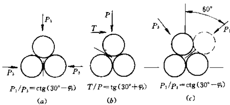
图 2-64 接触面的变化
