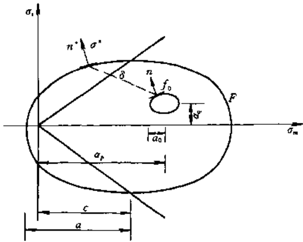
图 2-52 双椭圆模型
