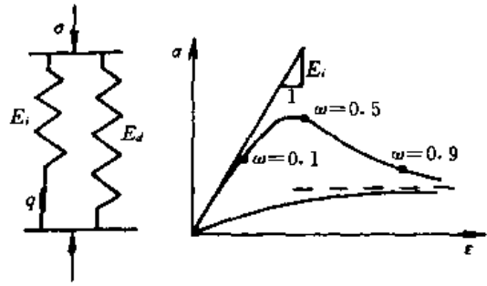
图 2-68 双弹簧模型
