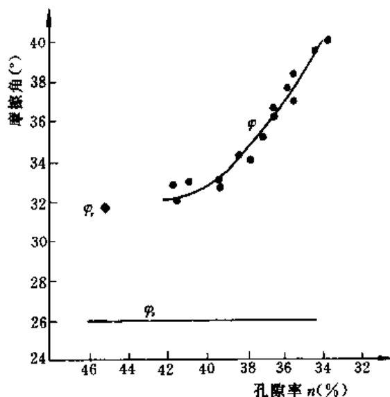
图 2-20 中砂摩擦角与起始孔隙率的关系
