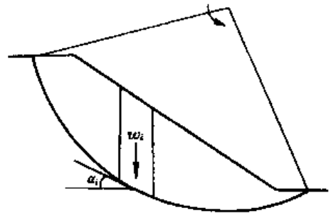
图 5-59 圆弧滑动面
