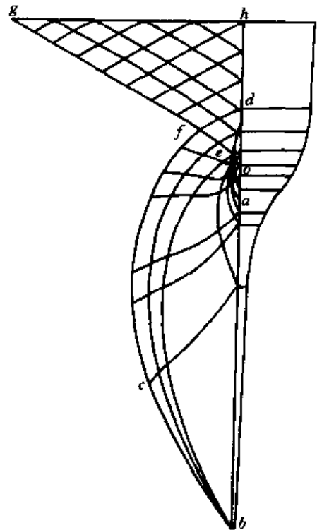
图 5-54 旋转运动墙
