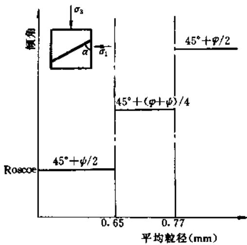
图 8-5 剪切带倾角
