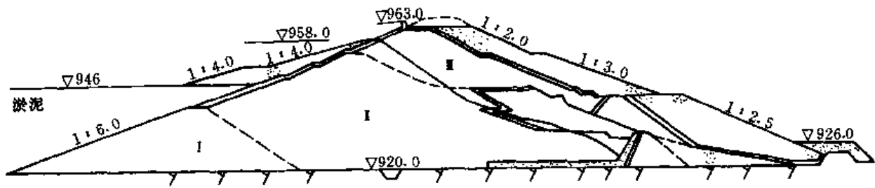
图 7-9 册田水库大坝断面
