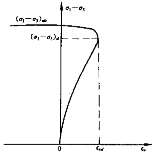
图 2-32 剪胀曲线
