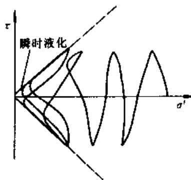
图 7-2 瞬时液化和循环活动性
