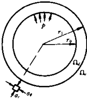
图 8-9 柱孔扩张
