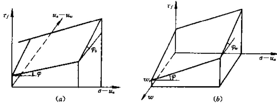
图 2-26 非饱和土强度
