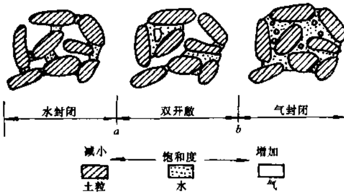
图 6-1 非饱和土三种含水状态
