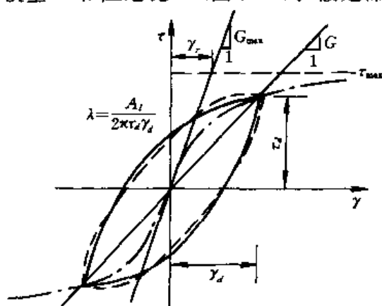
A_l 滞回圈面积 —— 实际滞回圈 - - - 等价椭圆 - - - 骨架曲线
