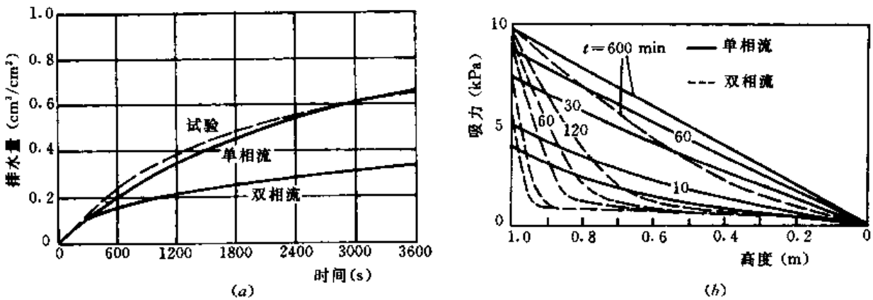
图 6-15 土柱排水
