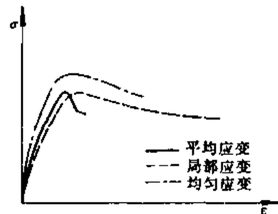
图 8-4 不同方法测定的应变
