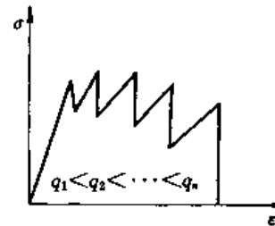
图 2-8 脆性破坏模型
