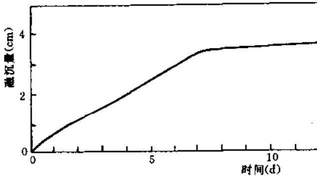
图 6-21 地面融沉过程线
