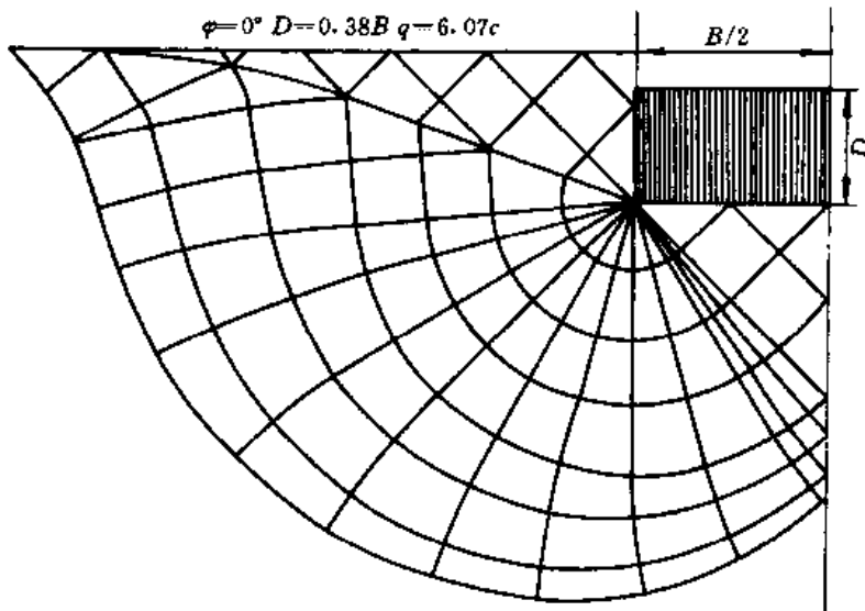
图 5-41 凝聚土算例
