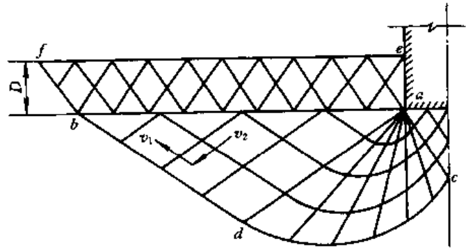
图 5-37 埋深地基的不连续解
